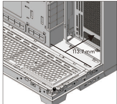
Clearance for side radiator (bracket reverse)/ 側邊散熱器支援尺寸(反裝)/Dégagement pour le radiateur latéral (support inversé)
