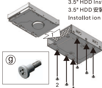
If space is needed, the hard drive cage can be removed/ 如有空間需求可將硬碟籠卸除/ Si de l'espace est nécessaire, la cage du disque dur p être retirée
