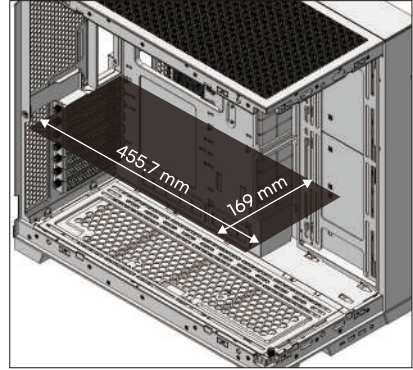
Clearance for upper position/上置模式空間/ Dégagement pour la position supérieure
