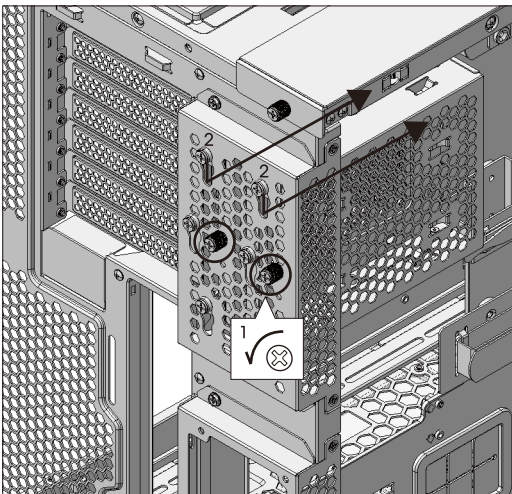
If space is needed, the hard drive cage can be removed/ 如有空間需求可將硬碟籠卸除/ Si de l'espace est nécessaire, la cage du disque dur p être retirée
