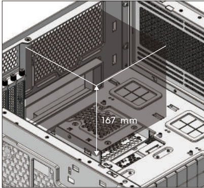
Clearance for lower position/下置模式空間/ Dégagement pour la position inférieure
