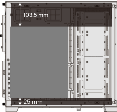
Clearance for side radiator/ 側邊散熱器支援尺寸/ Dégagement pour le radiateur latéral
