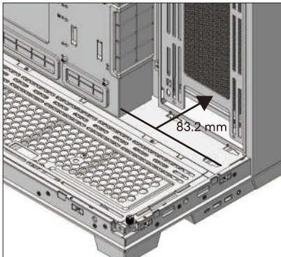
Clearance for side radiator/ 側邊散熱器支援尺寸/ Dégagement pour le radiateur latéral
